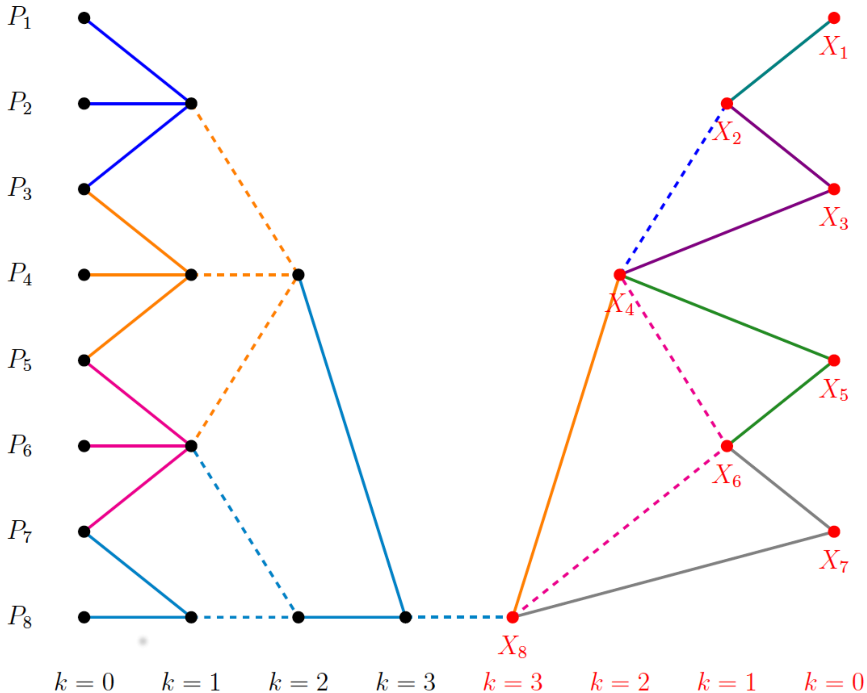
Abbildung 3.8: Datenabhängigkeiten beim Verfahren der zyklischen Reduktion für p = 8 ; ein \bullet repräsentiert in der Skizze die Daten B_i^{(k)} , C_i^{(k)} , D_i^{(k)} und E_i^{(k)}
