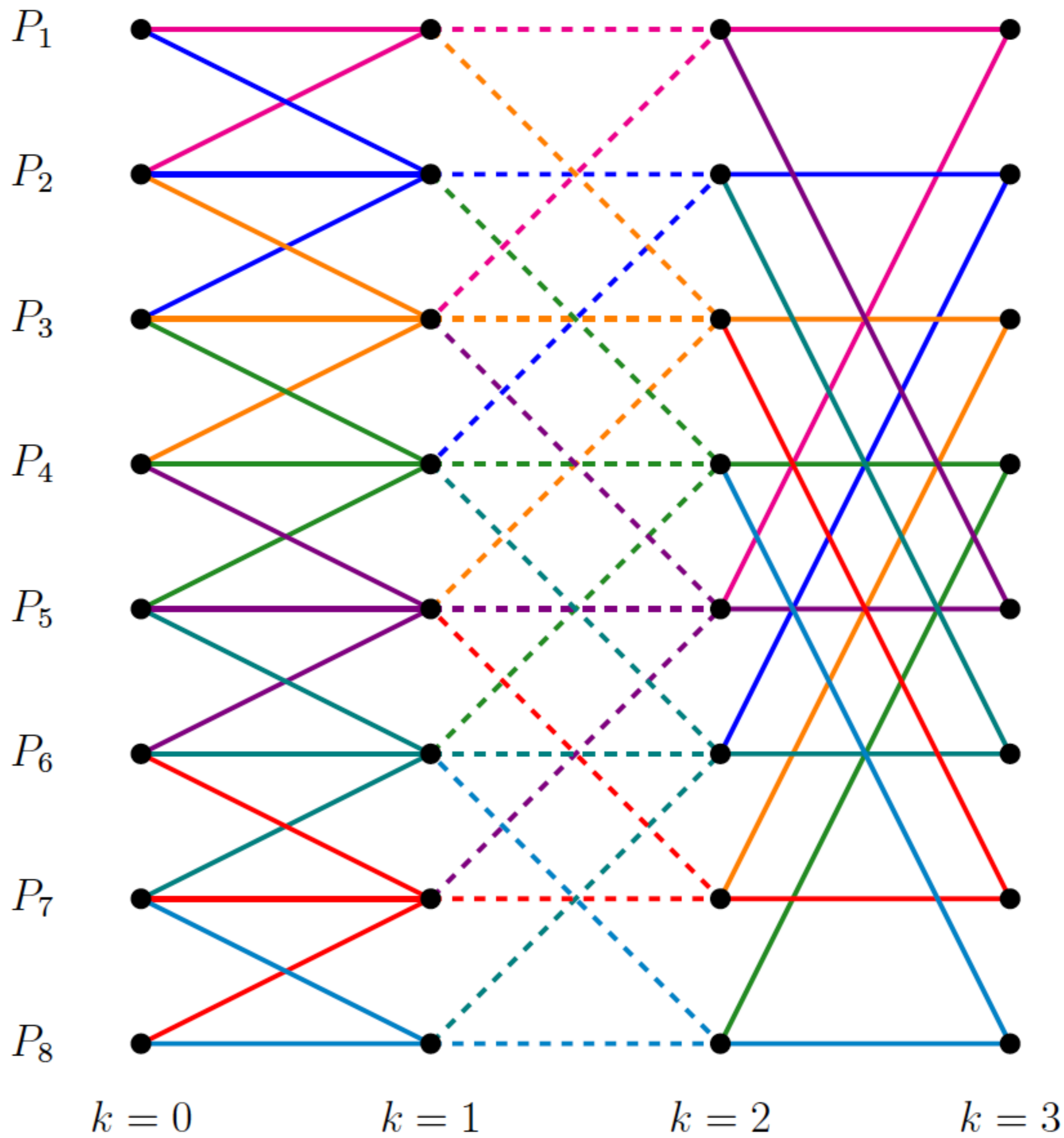
Abbildung 3.7: Datenabhängigkeiten beim rekursiven Verdoppeln für p = 8 ; ein \bullet repräsentiert in der Skizze die Daten B_i^{(k)} , C_i^{(k)} , D_i^{(k)} und E_i^{(k)}
